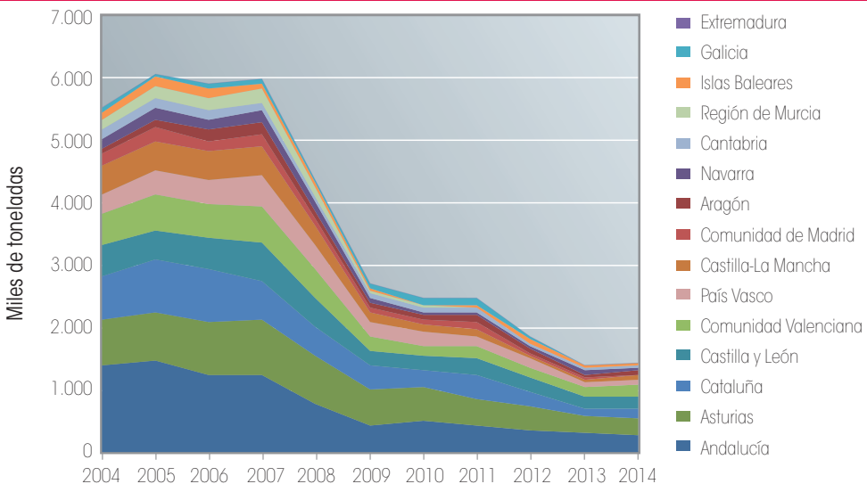
Gráfico 1. Evolución del consumo total en España de materias primas alternativas durante el periodo 2004-2014, por acumulación de consumos autonómicos (miles de toneladas).
