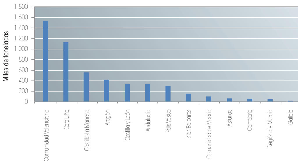
Gráfico 10. Emisiones de CO 2 evitadas en España por valorización energética en plantas cementeras durante el periodo 2004-2014 (miles de toneladas).
