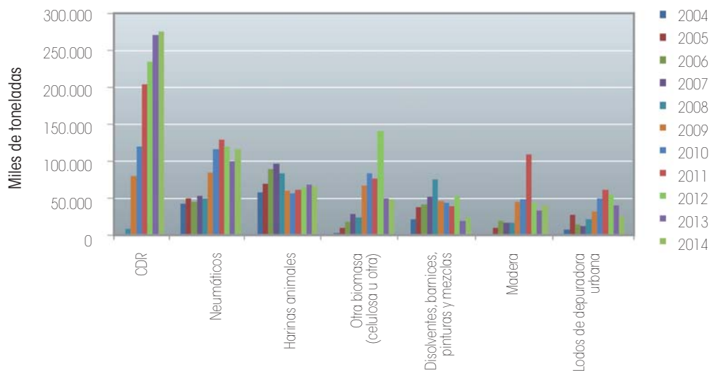
Gráfico 8. Evolución del consumo en España de combustibles alternativos durante el periodo 2004-2014 4 .
