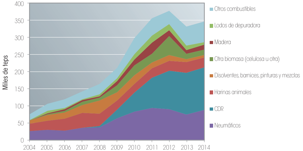
Gráfico 9. Evolución de la generación energética acumulada en España a partir de los diferentes tipos de combustibles alternativos los años del periodo 2004-2014 (miles de tep).
