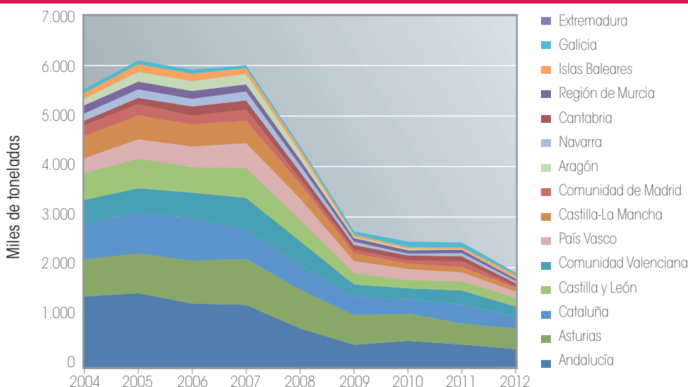
Gráfico 1. Evolución del consumo total en España de materias primas alternativas durante el periodo 2004-2012, por acumulación de consumos autonómicos.
