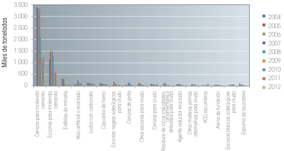
Gráfico 4. Evolución del consumo total en España de los diferentes tipos de materias primas alternativas (se incluyen únicamente aquellas con un consumo acumulado superior a 250.000 toneladas durante el periodo 2004-2012).
