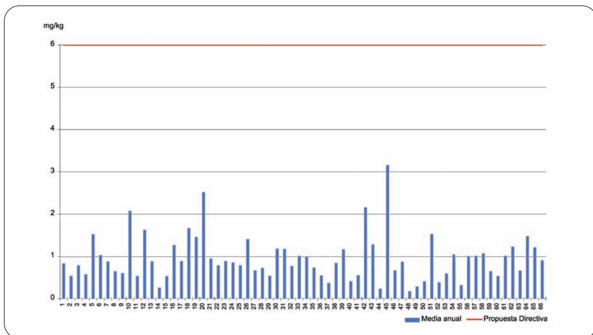
Figura 34. Contenido medio de PAH en los lodos de las diferentes EDAR del estudio
