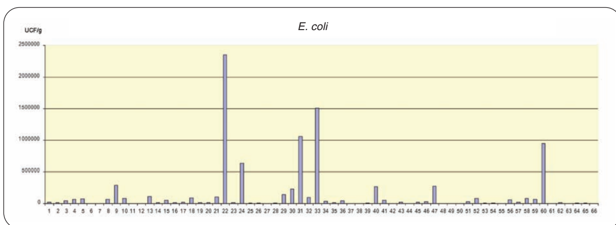
Figura 23. Concentración media de E. coli en los lodos de las diferentes EDAR del estudio
