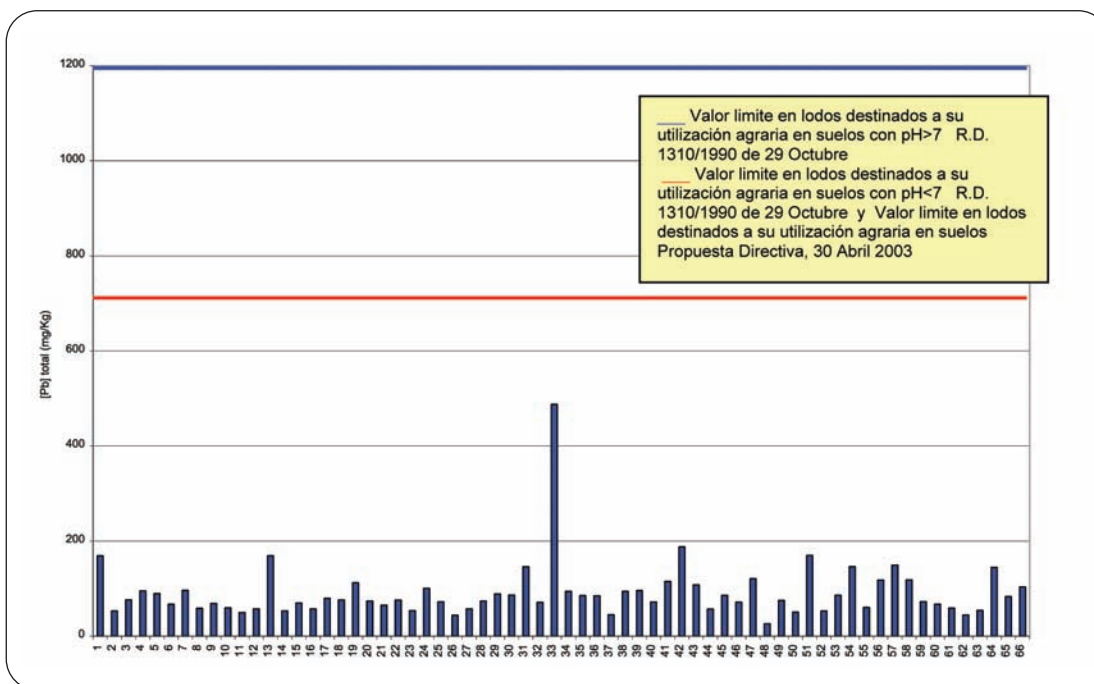
Figura 19. Concentración media de Pb en los lodos de las diferentes EDAR del estudio
