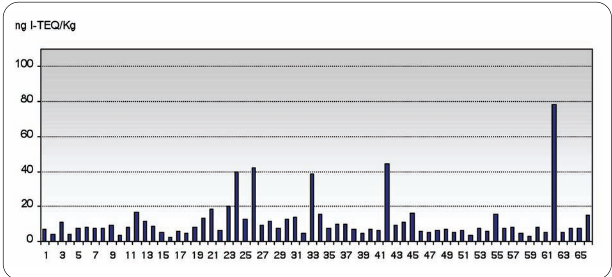
Figura 38. Contenido medio en PCDD/F en los lodos de las diferentes EDAR del estudio
