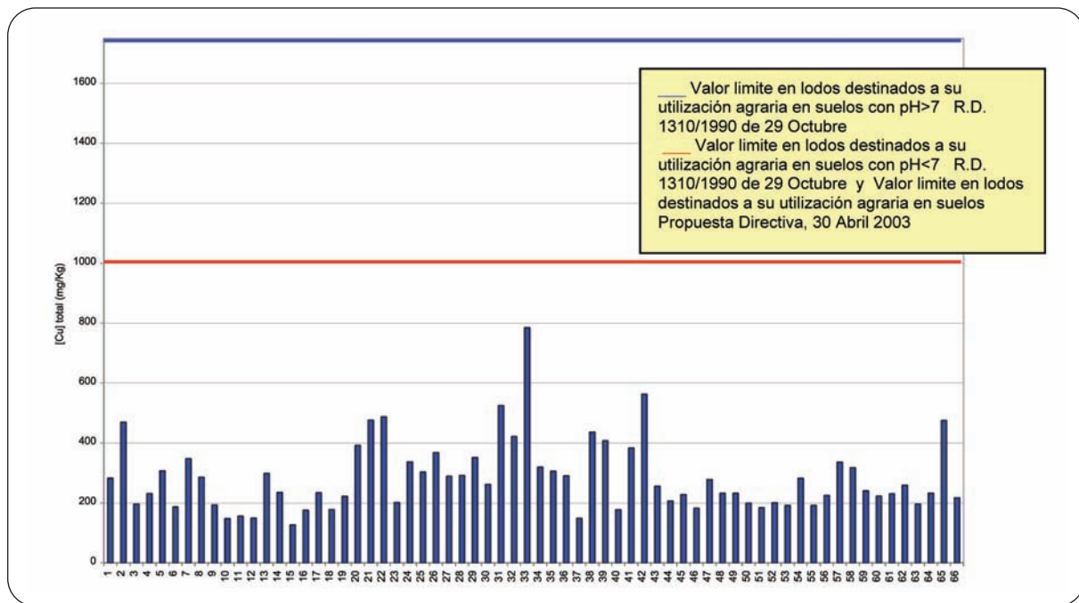
Figura 13. Concentración media de Cu en los lodos de las diferentes EDAR del estudio
