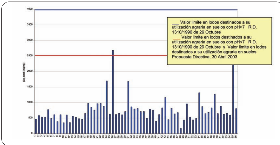
Figura 21. Concentración media de Zn en los lodos de las diferentes EDAR del estudio
