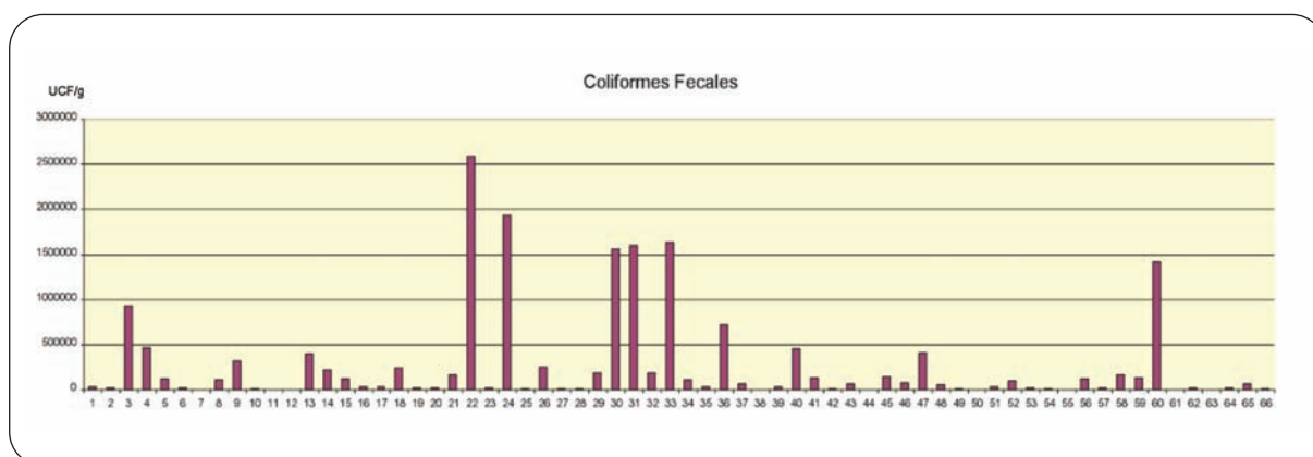
Figura 25. Concentración media de Coliformes fecales en los lodos de las diferentes EDAR del estudio
