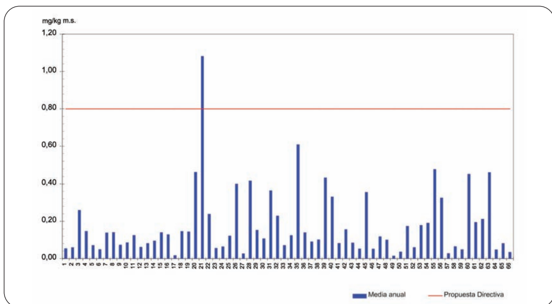
Figura 36. Contenido medio de PCB en los lodos de las diferentes EDAR del estudio
