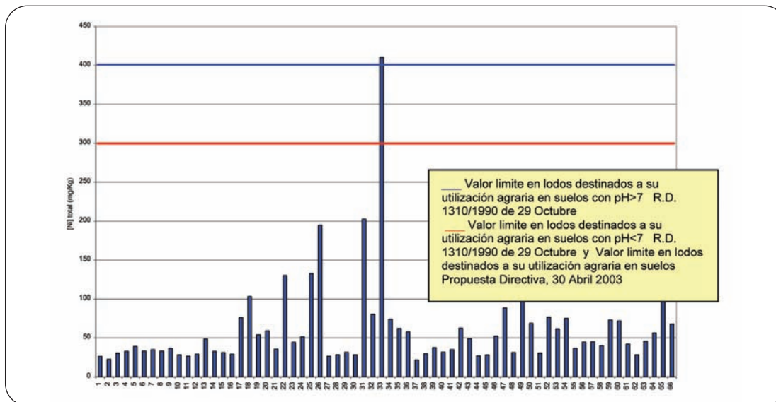
Figura 17. Concentración media de Ni en los lodos de las diferentes EDAR del estudio
