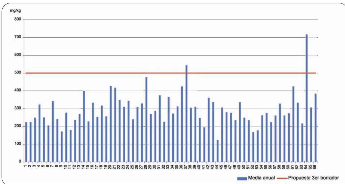
Figura 26. Contenido medio de AOX en los lodos de las diferentes EDAR del estudio
