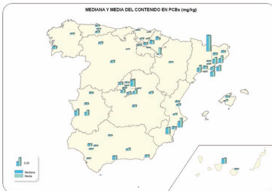
Figura 37. Distribución geográfica del contenido en PCB en los lodos de las diferentes EDAR del estudio
