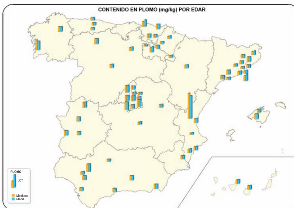
Figura 20. Distribución geográfica del contenido en Pb en los lodos de las diferentes EDAR del estudio
