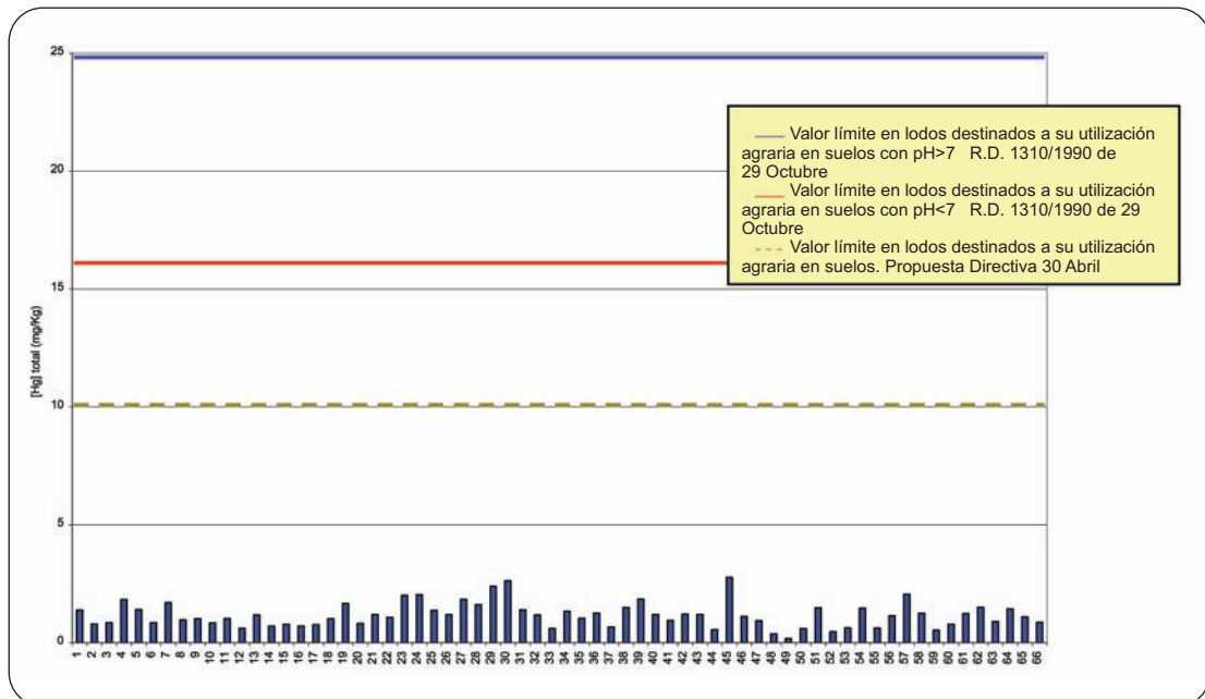
Figura 15. Concentración media de Hg en los lodos de las diferentes EDAR del estudio
