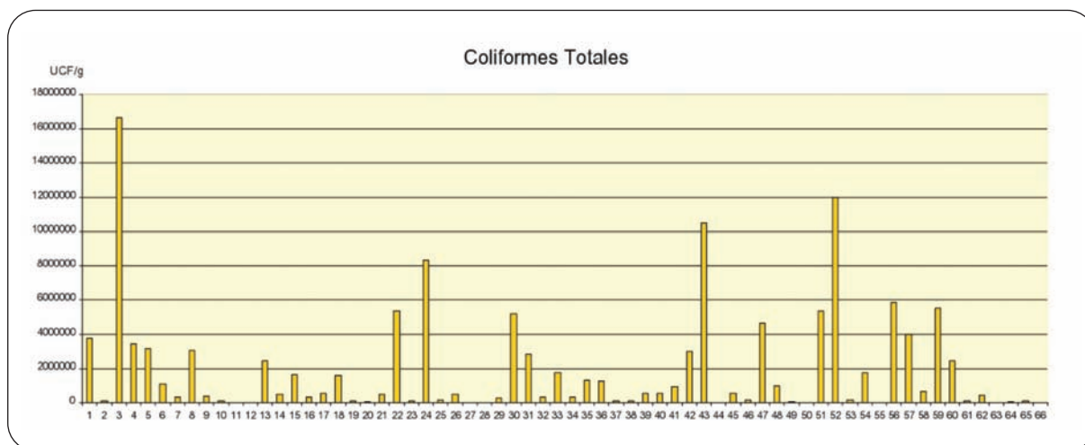
Figura 24. Concentración media de Coliformes Totales en los lodos de las diferentes EDAR del estudio
