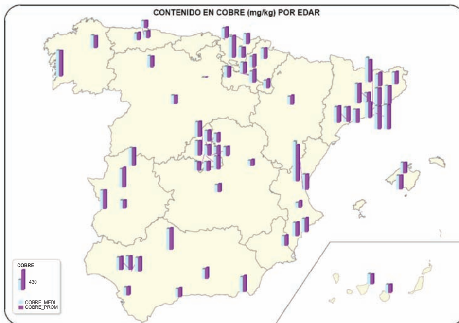
Figura 14. Distribución geográfica del contenido en Cu en los lodos de las diferentes EDAR del estudio
