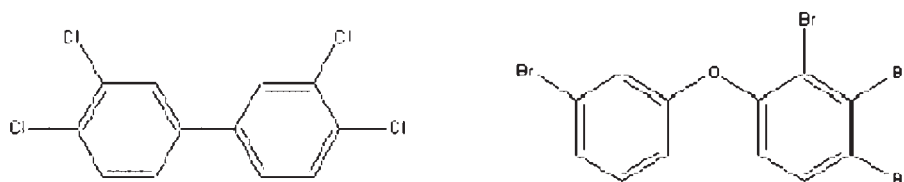
Estructura química de los PCBs (izq). Comparación con la estructura de los PBDEs (dcha)
