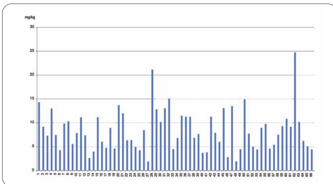
Figura 28. Contenido medio de DEHP en los lodos de las diferentes EDAR del estudio
