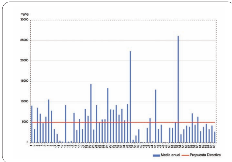
Figura 32. Contenido medio de LAS en los lodos de las diferentes EDAR del estudio
