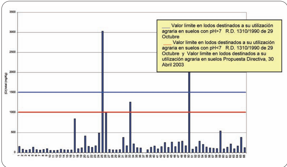
Figura 11. Concentración media de Cr total en los lodos de las diferentes EDAR del estudio
