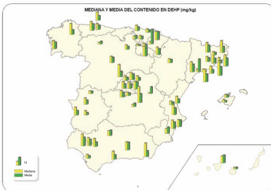
Figura 29. Distribución geográfica del contenido en DEHP en los lodos de las diferentes EDAR del estudio
