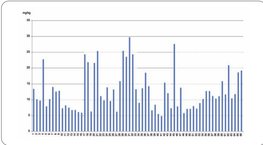
Figura 30. Contenido medio de NPE en los lodos de las diferentes EDAR del estudio
