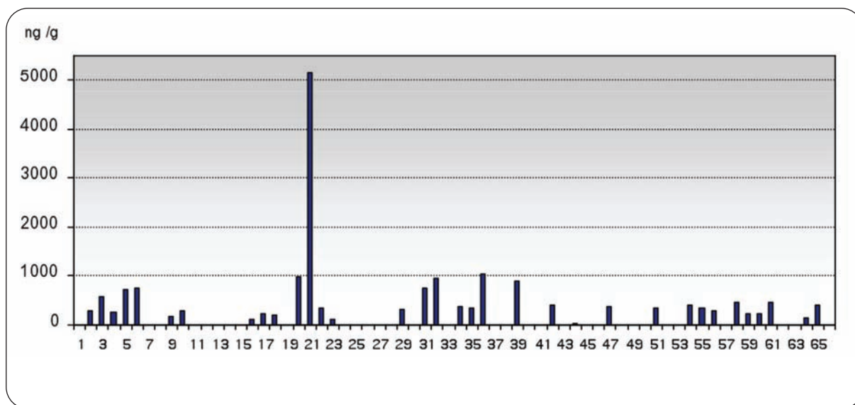
Figura 40. Contenido medio en PBDE en los lodos de las diferentes EDAR del estudio
