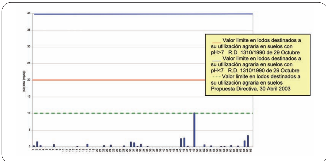
Figura 9. Concentración media de Cd en los lodos de las diferentes EDAR del estudio
