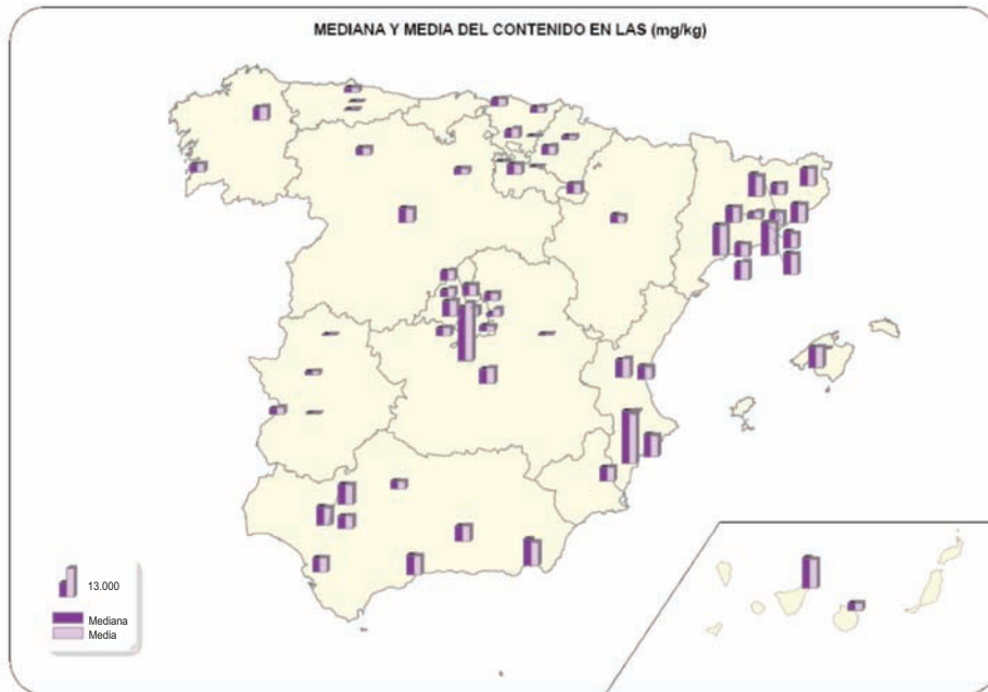
Figura 33. Distribución geográfica del contenido en LAS en los lodos de las diferentes EDAR del estudio
