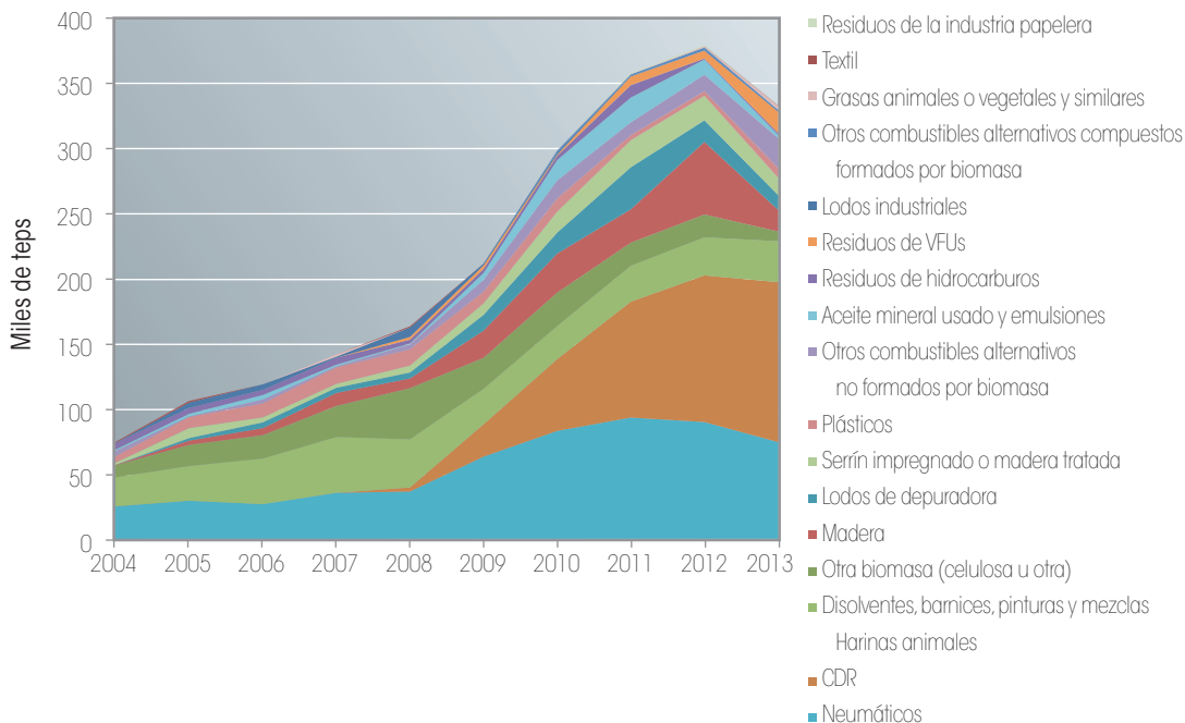
Gráfico 9. Evolución de la generación energética acumulada en España a partir de los diferentes tipos de combustibles alternativos, periodo 2004-2013
