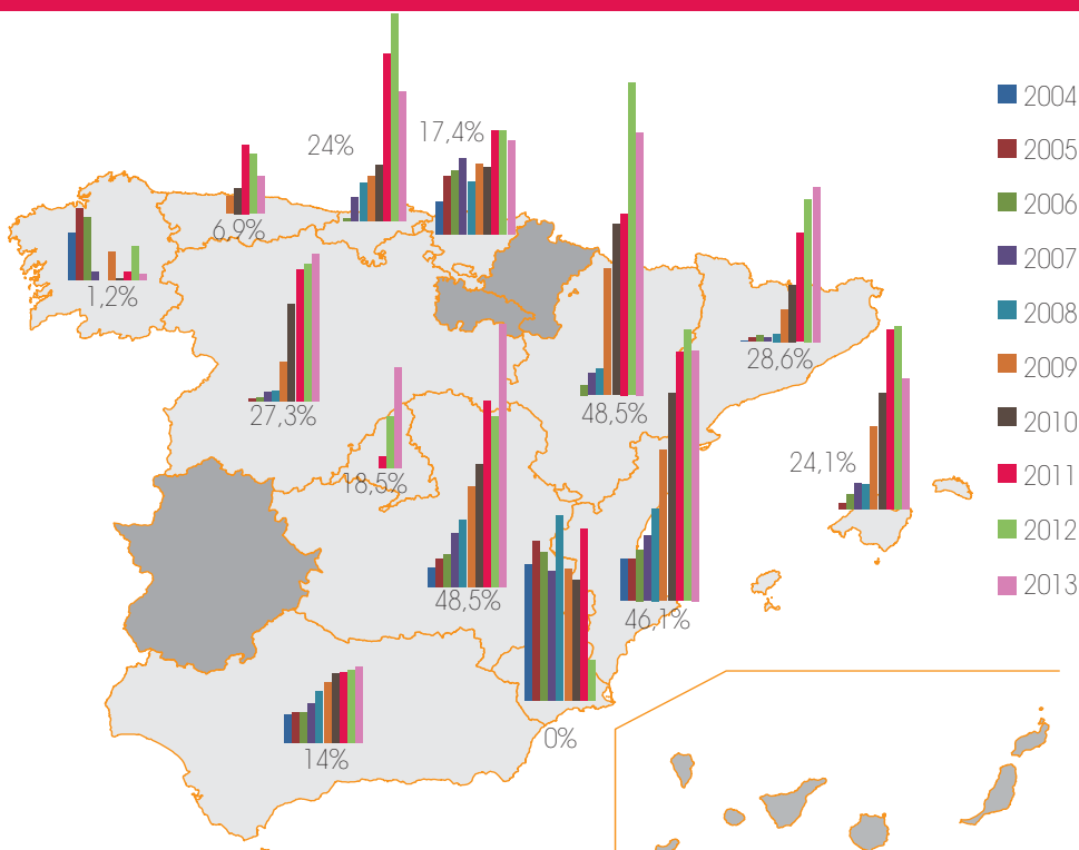
Figura 5. Porcentaje de sustitución energética de combustibles alternativos por comunidad autónoma (periodo 2004-2013).
