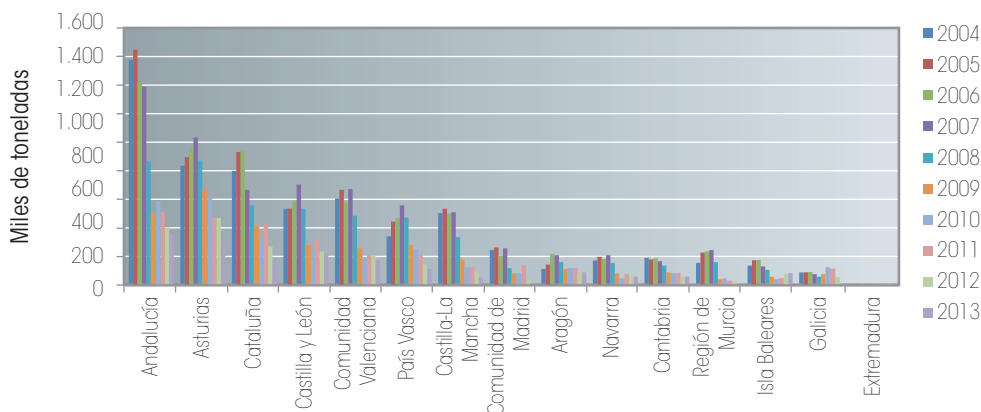
Gráfico 3. Consumos totales anuales de materias primas alternativas por comunidades autónomas durante el periodo 2004-2013.
