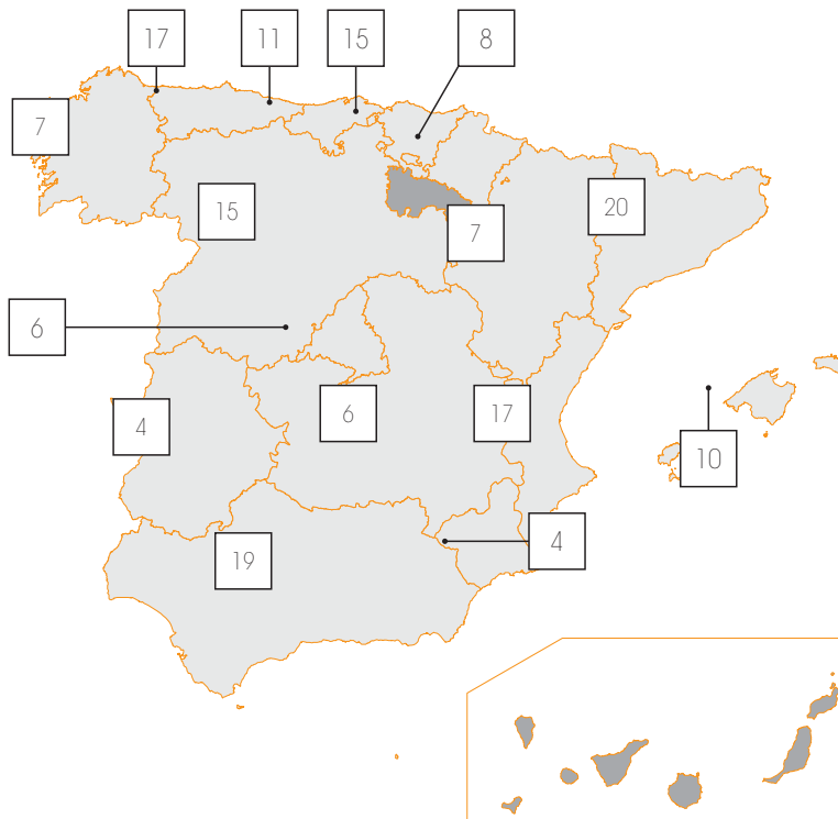
Figura 3. Número de tipologías de materias primas alternativas consumidas por comunidades autónomas (periodo 2004-2013).
