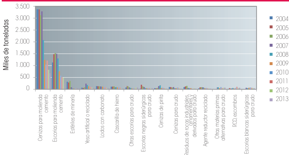
Gráfico 4. Evolución del consumo total en España de los diferentes tipos de materias primas alternativas (se incluyen únicamente aquellas con un consumo acumulado superior a 300.000 toneladas durante el periodo 2004-2013).
