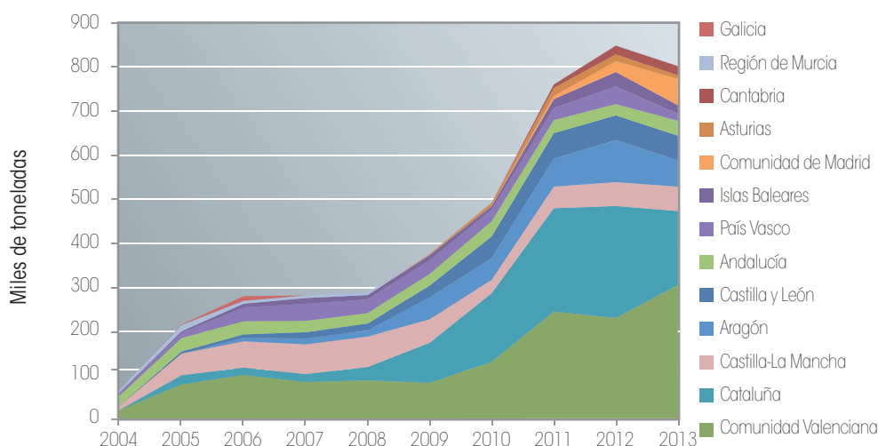
Gráfico 10. Evolución de las emisiones de CO 2 evitadas en España por valorización energética en plantas cementeras durante el periodo 2004-2013.
