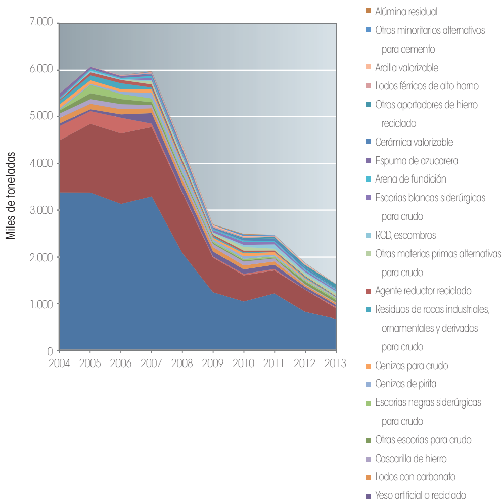
Gráfico 2. Evolución del consumo total en España de materias primas alternativas, periodo 2004-2013, según tipologías de materias primas (miles de toneladas).
