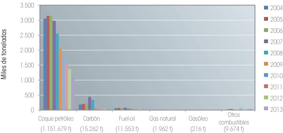
Gráfico 6. Evolución del consumo total en España de combustibles tradicionales durante el periodo 2004-2013.
