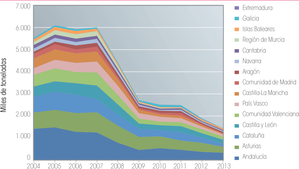
Gráfico 1. Evolución del consumo total en España de materias primas alternativas, periodo 2004-2013, por acumulación de consumos autonómicos.
