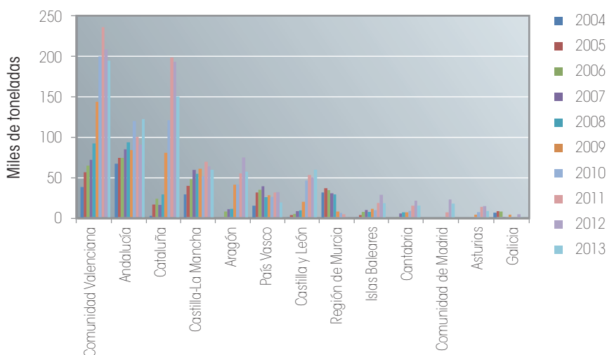
Gráfico 7. Consumo de combustibles alternativos por comunidades autónomas durante los años del periodo 2004-2013 (miles de toneladas).
