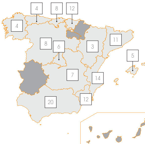
Gráfico 7. Consumo de combustibles alternativos por comunidades autónomas durante los años del periodo 2004-2013 (miles de toneladas).
