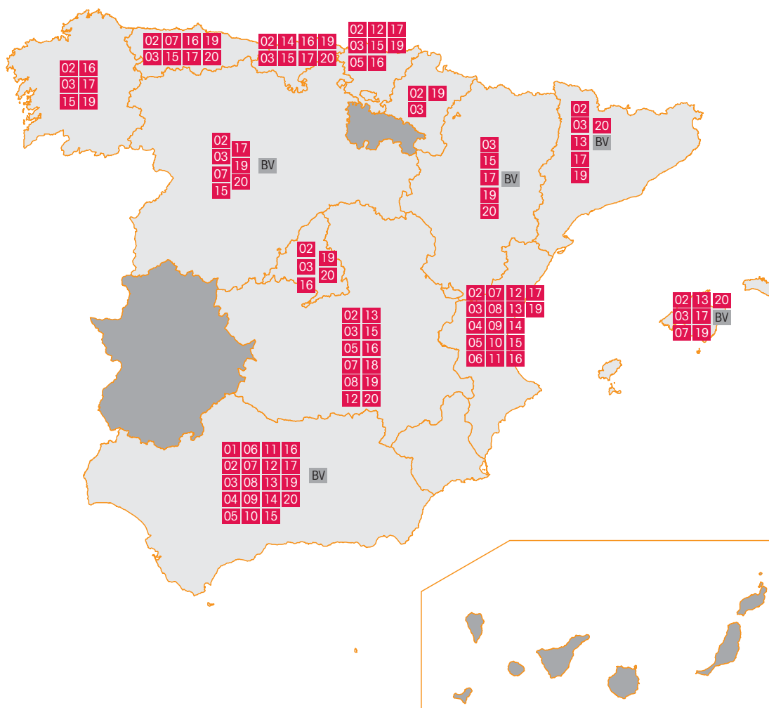
Figura 1. Residuos autorizados, por comunidades autónomas, para valorización energética en fábricas de cemento.
