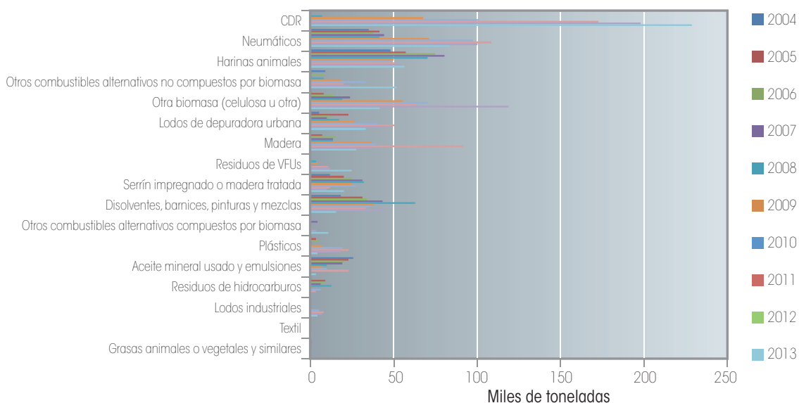
Gráfico 8. Evolución del consumo en España de combustibles alternativos durante el periodo 2004-2013.
